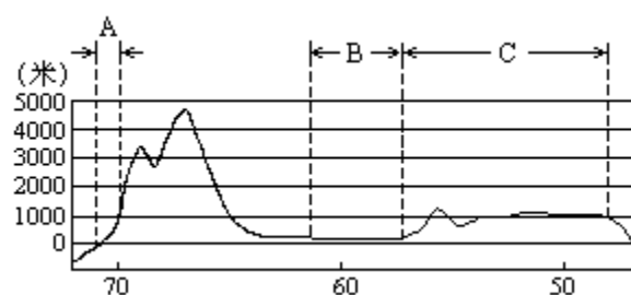
沿南回归线地形剖面图
