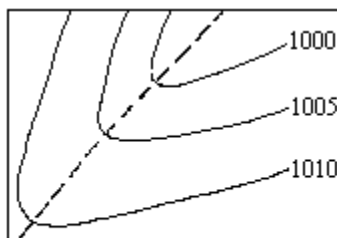
北半球中纬某地气压分布图 （单位：百帕）
